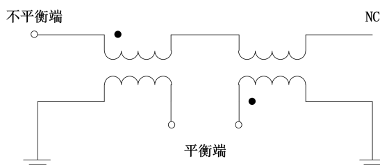
YLBL-16-E6-D产品原理图
